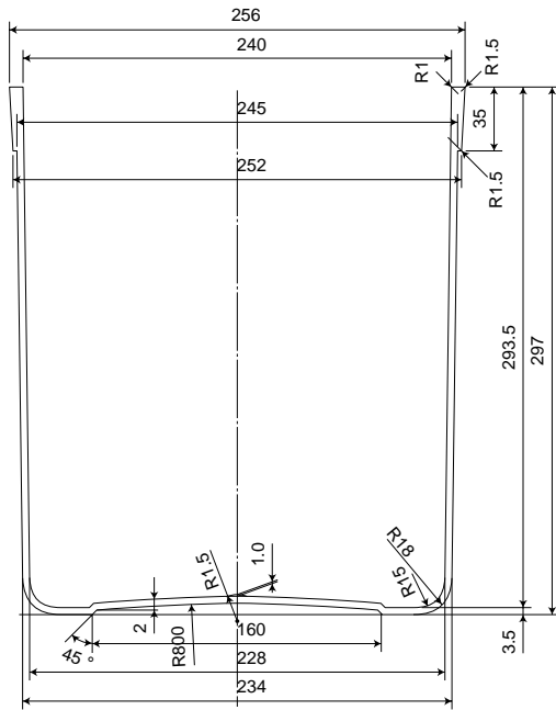
外形寸法図 NF-2
